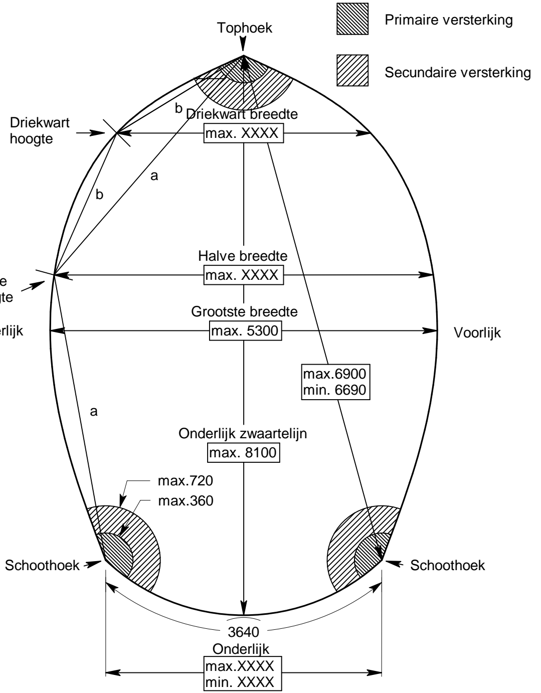
Maatvoering Regenboog Genua en Spinnaker
